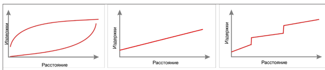
Рис. 1. Типы изменения затрат на авиаперевозки в зависимости от расстояния (слева направо – нелинейная, линейная, многофакторная)
