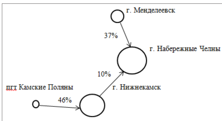
Рис. 1. Схема замещающих маятниковых миграций в агломерации Набережных Челнов.
